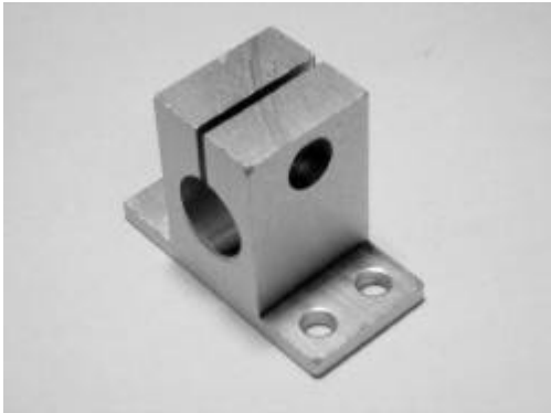
Montagebock aus Aluminium zur Aufbau-Montage von Wegaufnehmern
