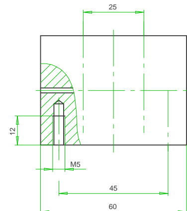
MB 25 Montageblock für Wegaufnehmer Ø25 mm, AlMgSi 0.5
